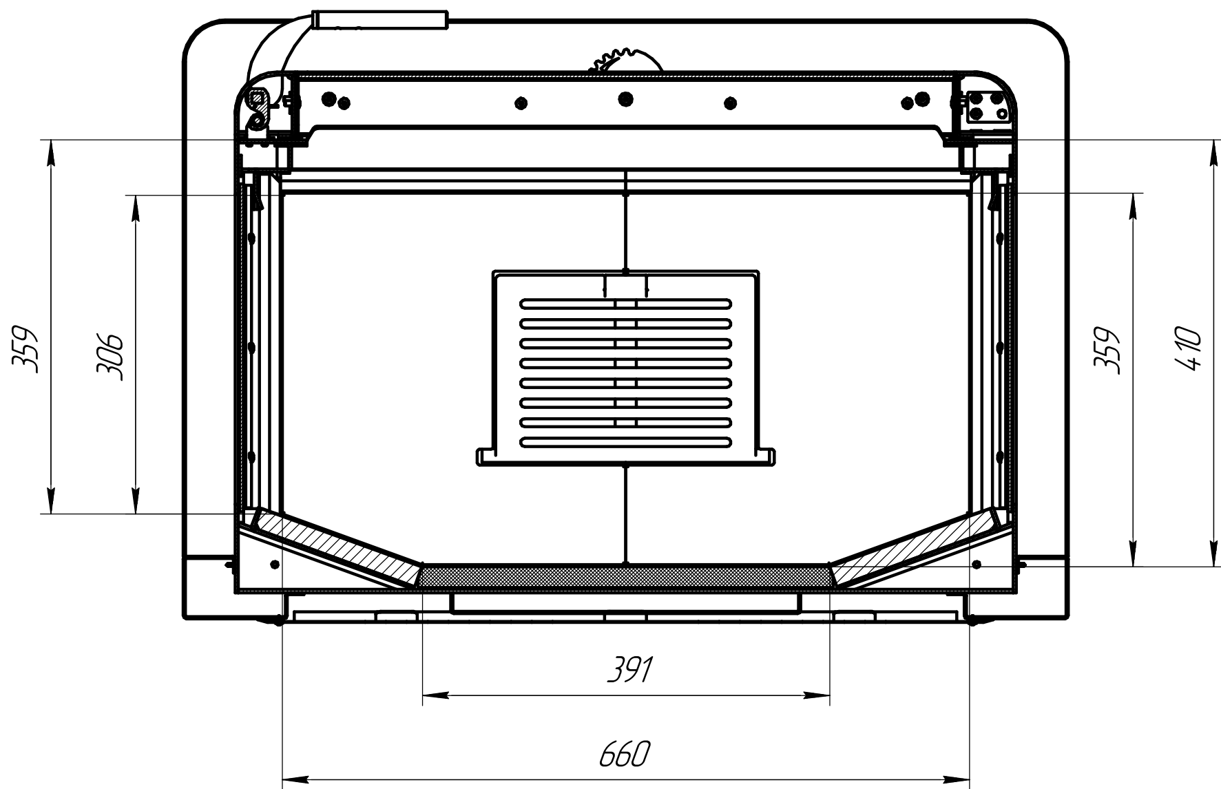
Б-Б(1:5)
